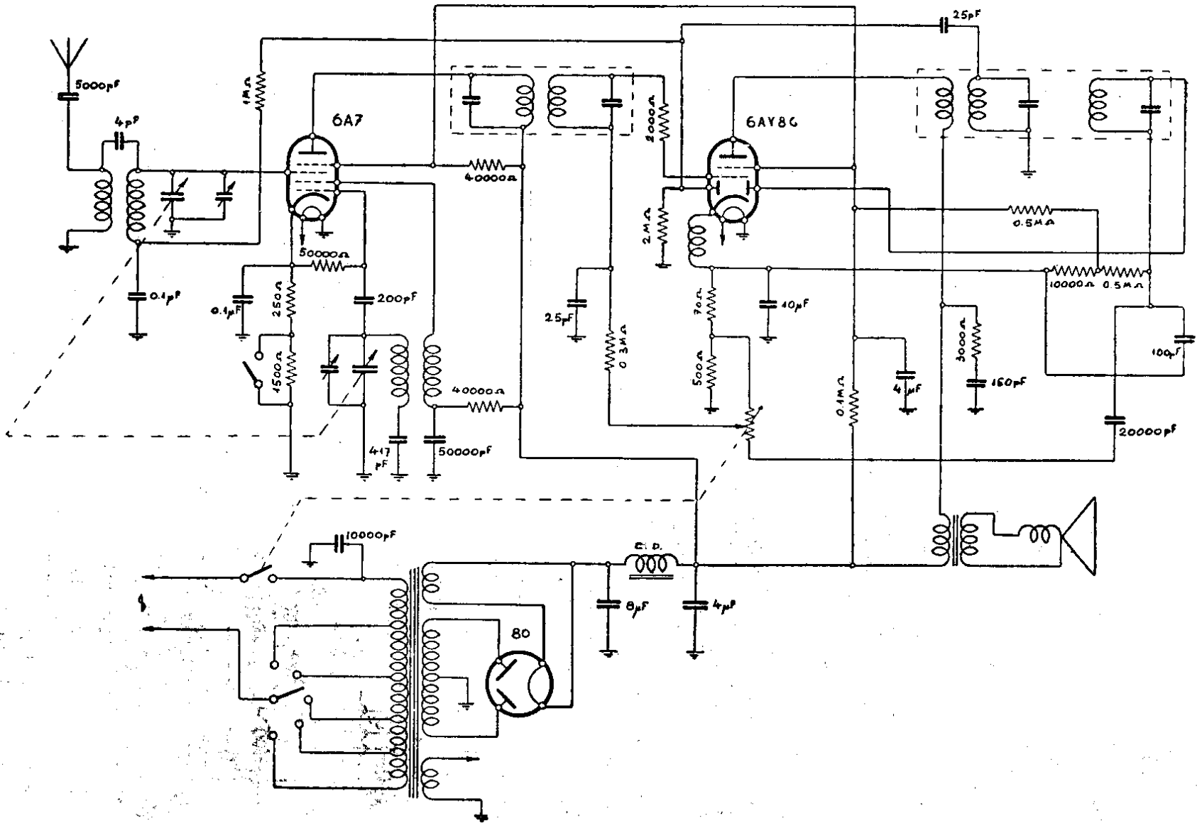
RADIO SAFAR. — Mod. « Roma ». — Media frequenza: 470 kHz. (Per i particolari e l'armamento descritto in Moderna Supereterodina, 5ª ediz.)
